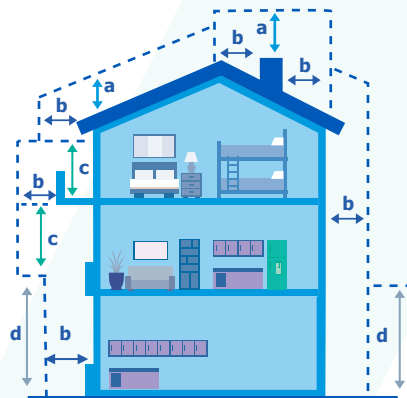
Figura 13.10.1.a. Distancias de seguridad en zonas con construcciones
